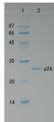
図1 ポリアクリルアミドゲルによる HIV-1 p24 タンパク質の電気泳動
